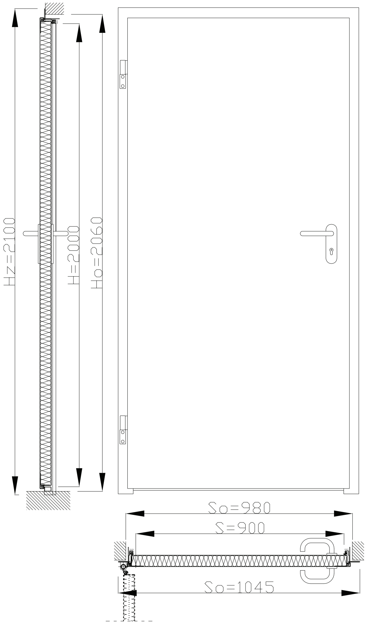
Rysunek techniczny drzwi ECO
